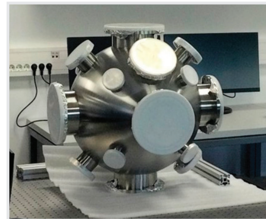
Vakuumska komora u kojoj atome stroncija hladimo pomoću lasera gotovo do apsolutne nule.
